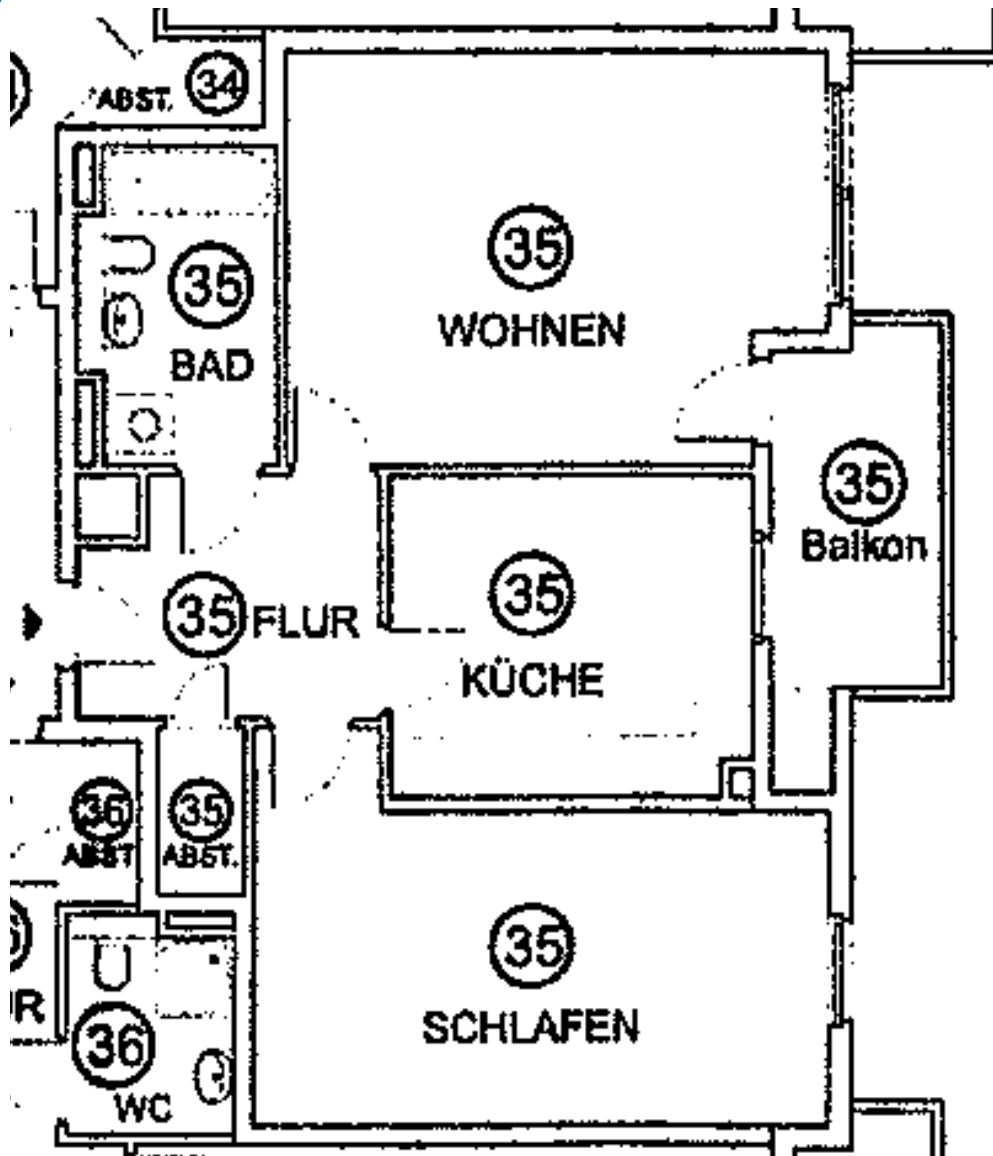
1. Obergeschoss (Nr. 35)
